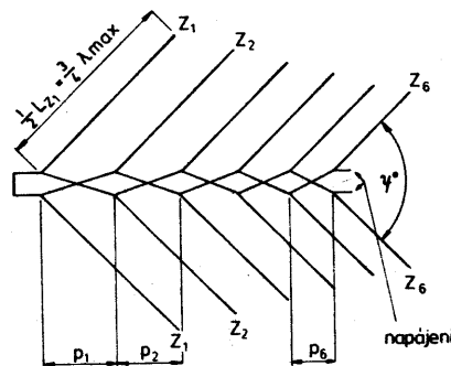
Obr. 5. Logaritmicko-periodická dipólová anténa s prvky ve tvaru V má zvýšené směrové účinky na lichých harmonických kmitočtech ( 3f, 5f, \dots ). Optimální úhel \psi pro 3f je 115^\circ
